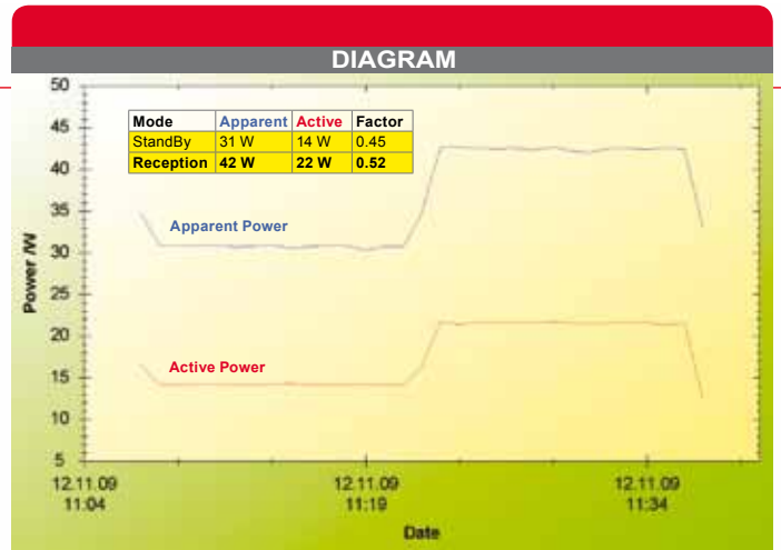
前15分钟:待机。第二个15分钟:第一分钟接收机接通电源,接下来的14分钟是包括切换频道、录像以及播放等等在内的动态使用。
